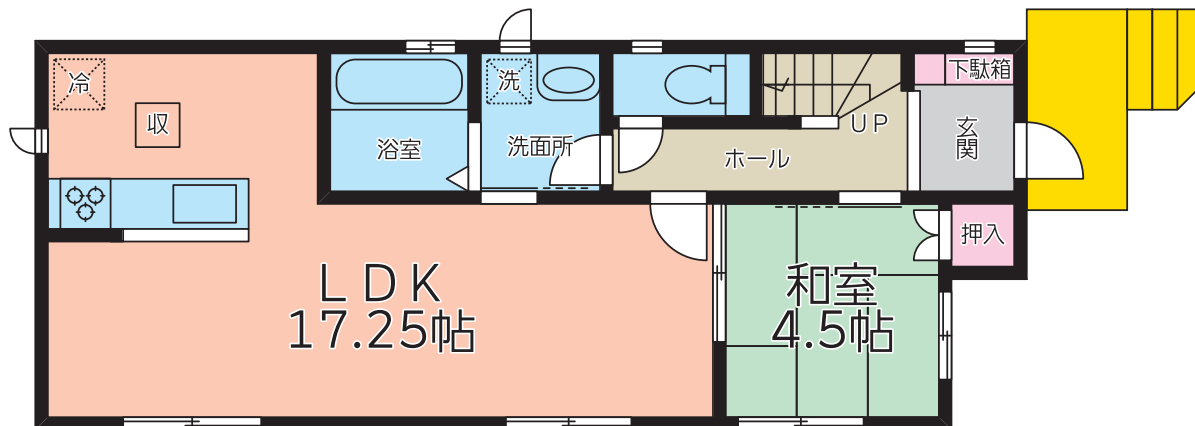
1階平面図:52.18㎡(15.78坪)
